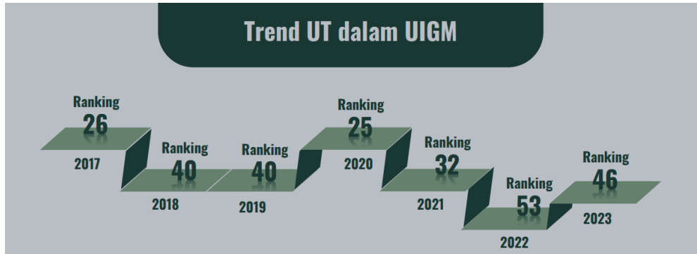
Gambar 46. Skor UT
